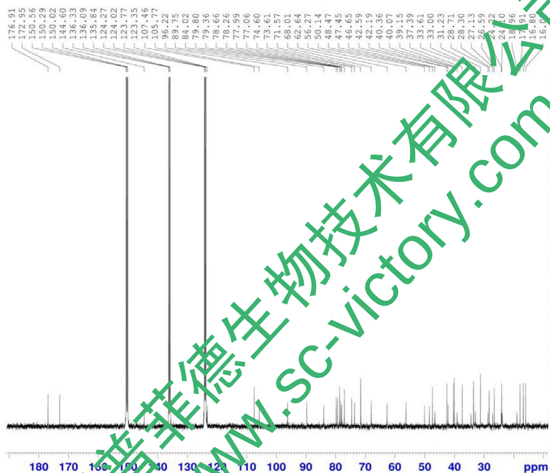
^{13}\text{C} -NMR 图
